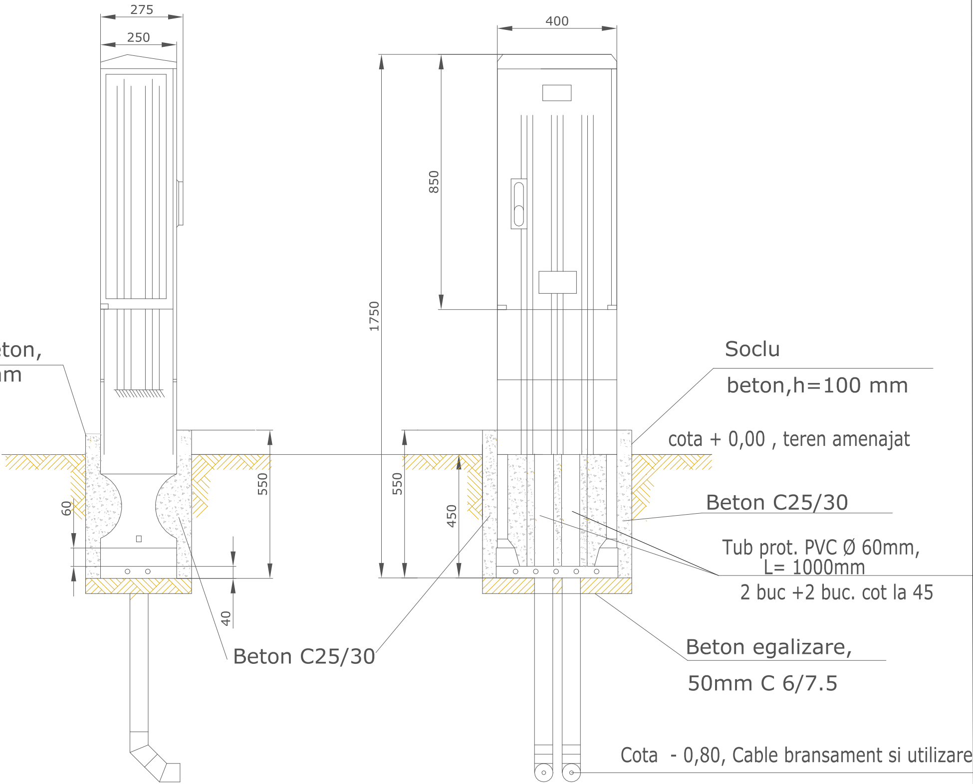
Vedere laterala
